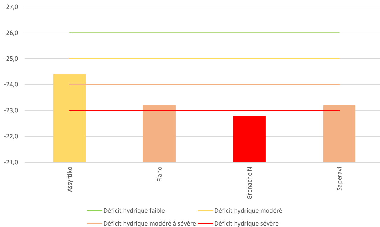
Analyses du \delta^{13}C saison 2024
