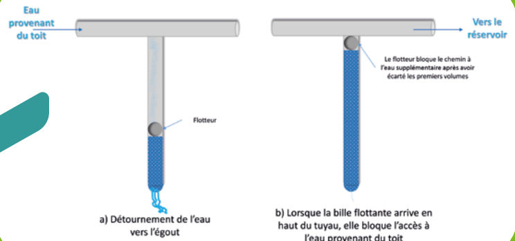
Figure 6 : disconnecteur
