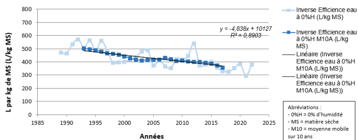
Figure 10 : Evolution de l'inverse de l'efficience de l'eau apportée chez le maïs
