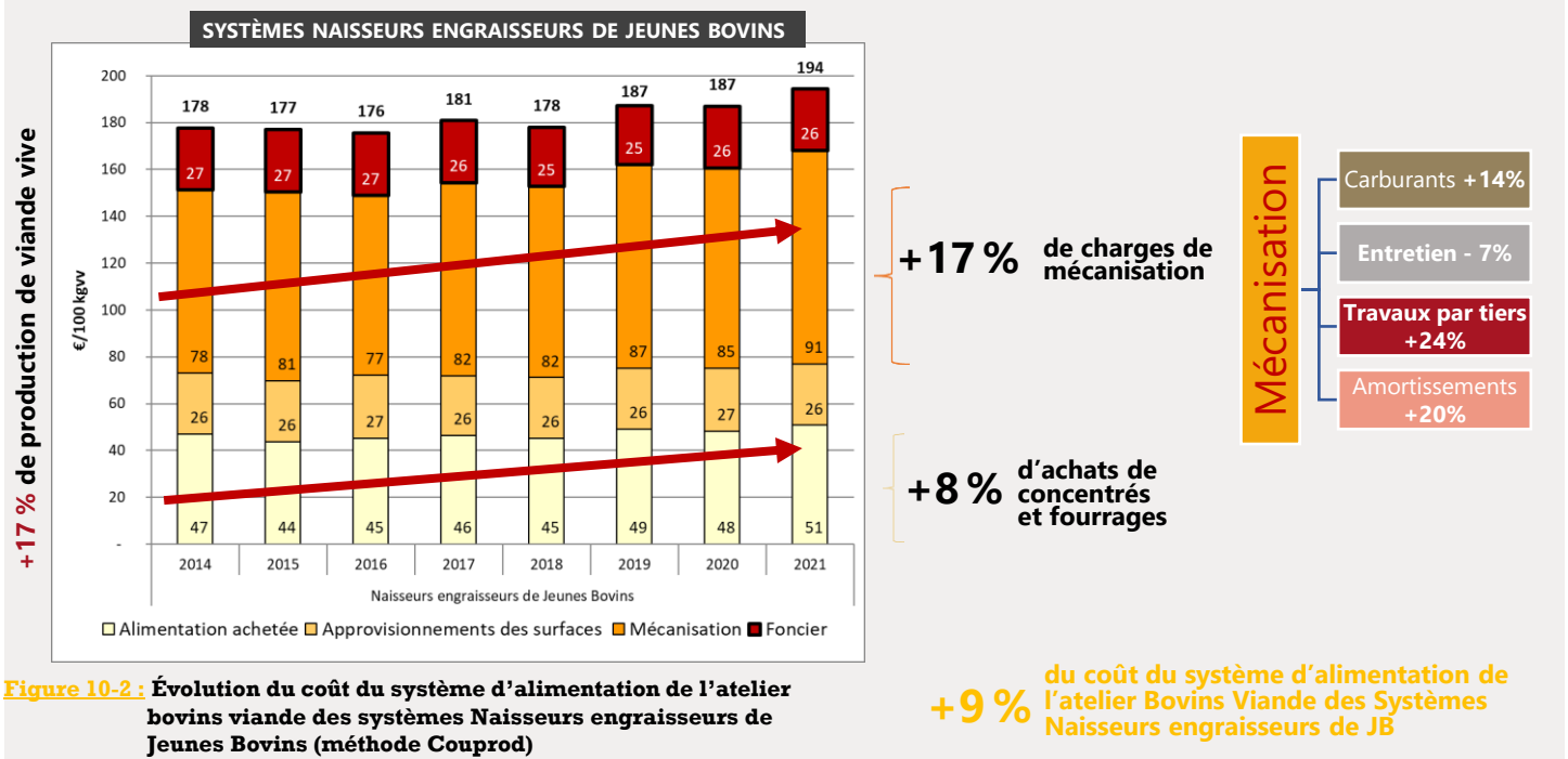
Figure 10-1 : Évolution du coût du système d'alimentation de l'atelier bovins viande des systèmes Naisseurs et Naisseurs engraisseurs de bœufs (méthode Couprod)
