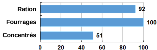
Autonomie massique (%)
