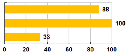
Autonomie protéique (%)
